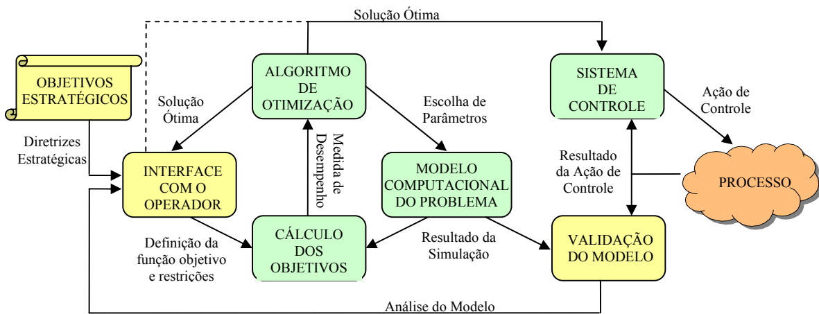
Fig.2 – Diagrama da Integração On-line de um Sistema de Otimização Fonte: Adaptado de TAKAHASHI, R. Otimização escalar e vetorial . Belo Horizonte: UFMG, Departamento de Matemática, Curso de verão, 2003.
